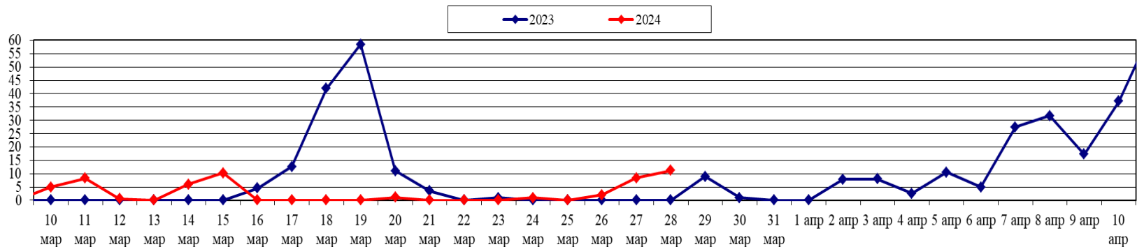
Площадь ландшафтных пожаров (2023-2024 гг. март-апрель)
