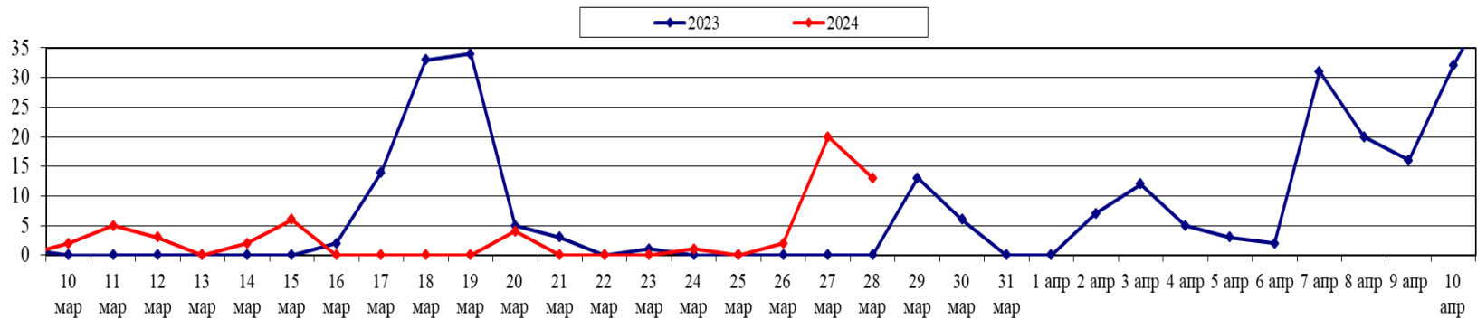
Количество ландшафтных пожаров (2023-2024 гг. март-апрель)
