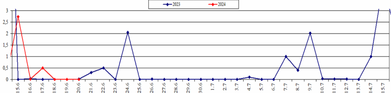
Площадь ландшафтных пожаров (2023-2024 гг. июнь - июль)
