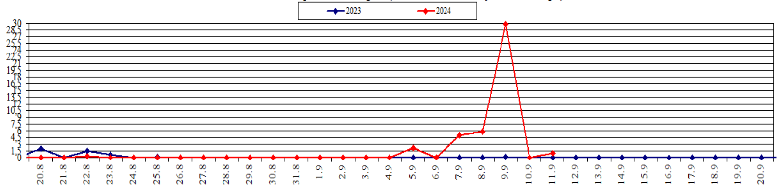
Площадь ландшафтных пожаров (2023-2024 гг. август - сентябрь)
