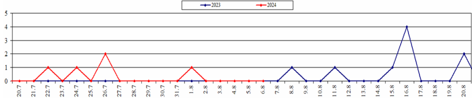
Площадь ландшафтных пожаров (2023-2024 гг. июль-август)
