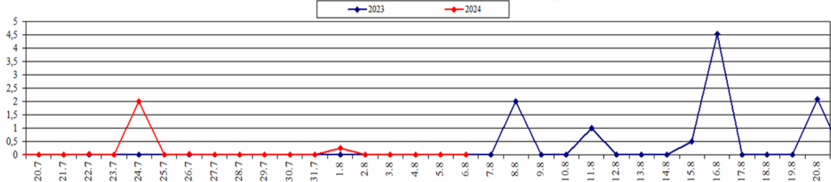
Площадь ландшафтных пожаров (2023-2024 гг. июль-август)
