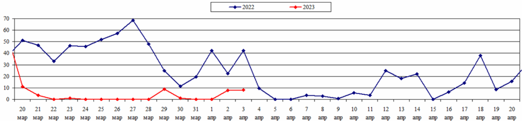
Площадь ландшафтных пожаров (2022-2023 гг., март - апрель)
