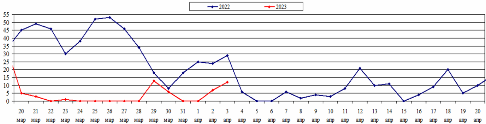
Количество ландшафтных пожаров (2022-2023 гг., март - апрель)
