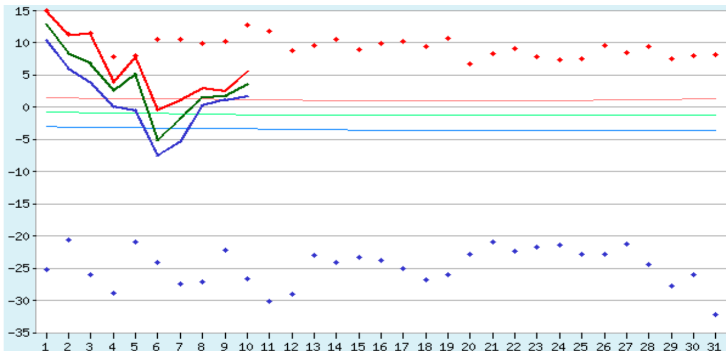
Температура воздуха в Калининграде. Январь 2023 г.
