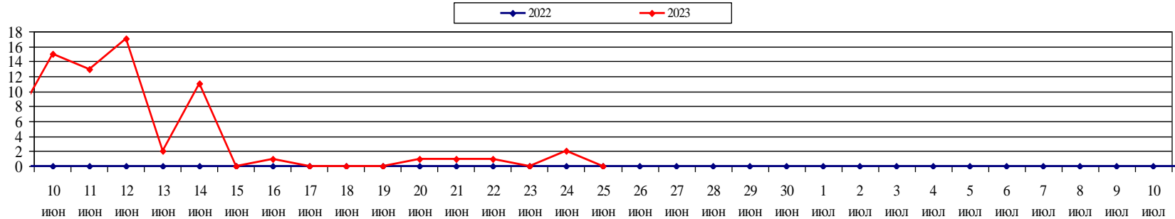
Количество ландшафтных пожаров (2022-2023 гг. июнь-июль)
