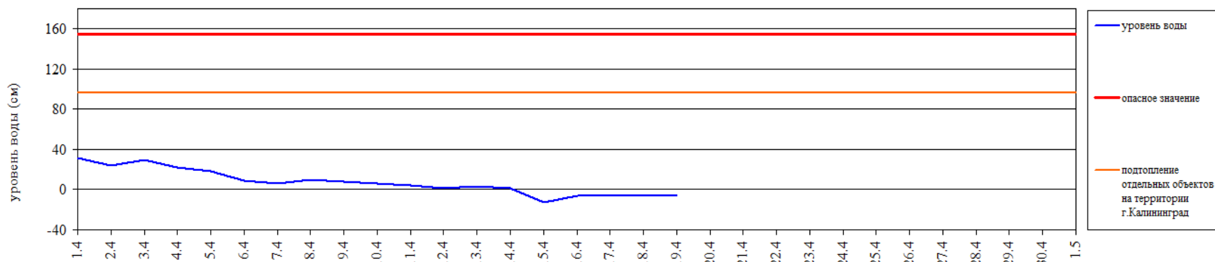
Уровень воды в р. Преголя относительно "0" поста МШК (г. Калининград)
