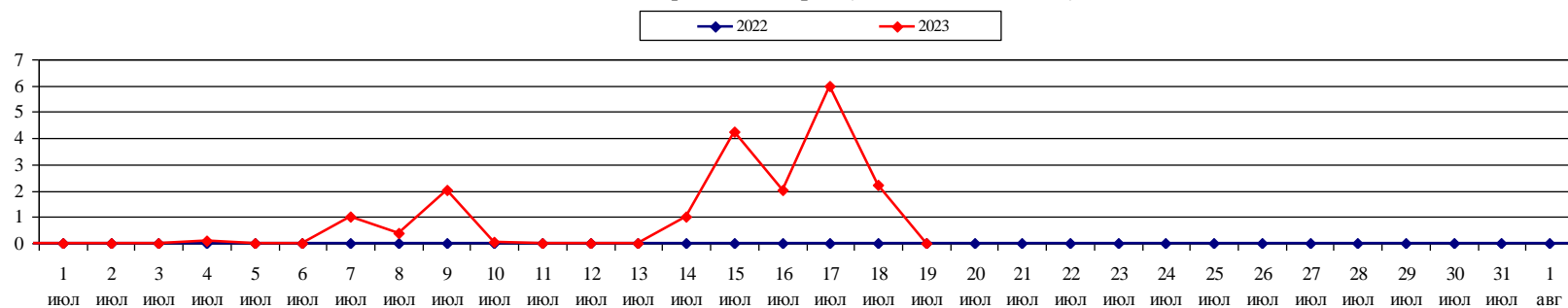
Площадь ландшафтных пожаров (2022-2023 гг. июль)
