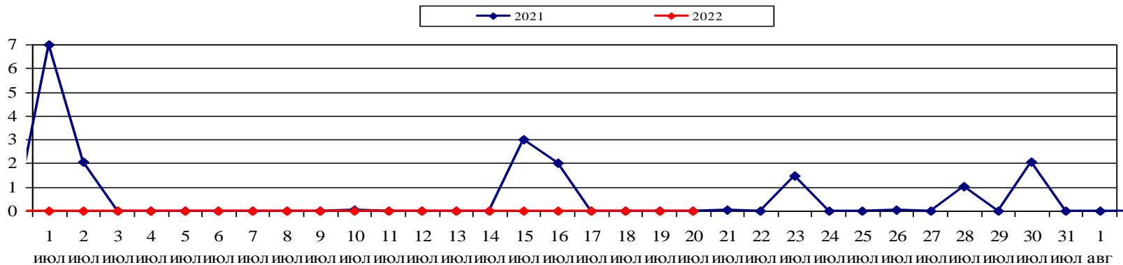
Площадь ландшафтных пожаров (2021-2022 гг., июль)
