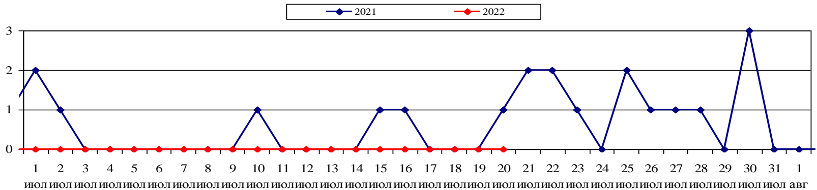
Количество ландшафтных пожаров (2021-2022 гг., июль)
