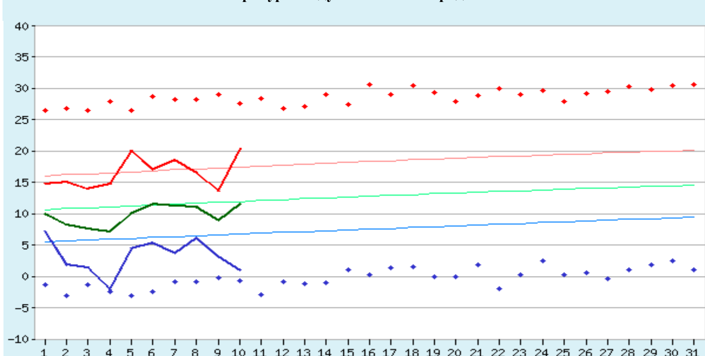
Температура воздуха в Калининграде. Май 2022 г.
