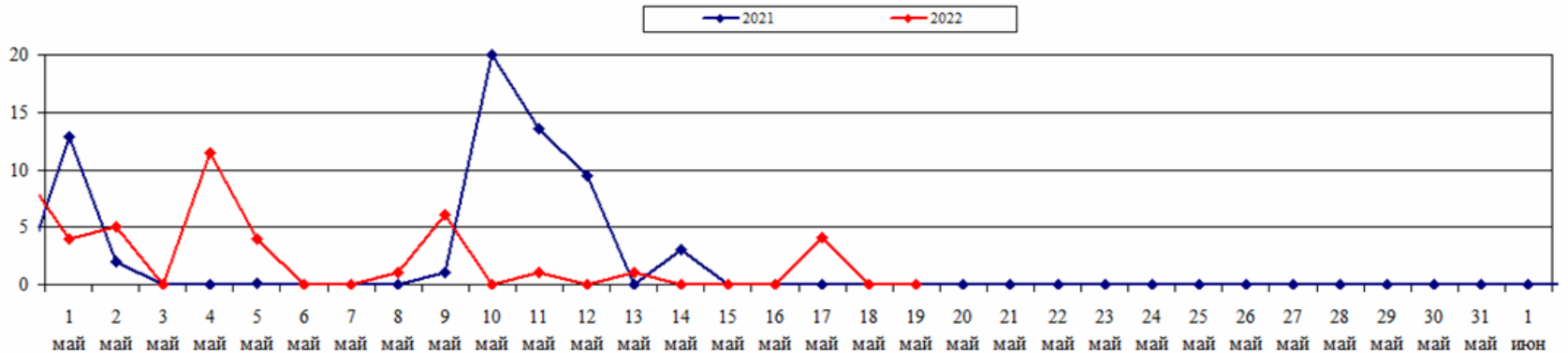
Площадь ландшафтных пожаров (2021-2022 гг., апрель - май)
