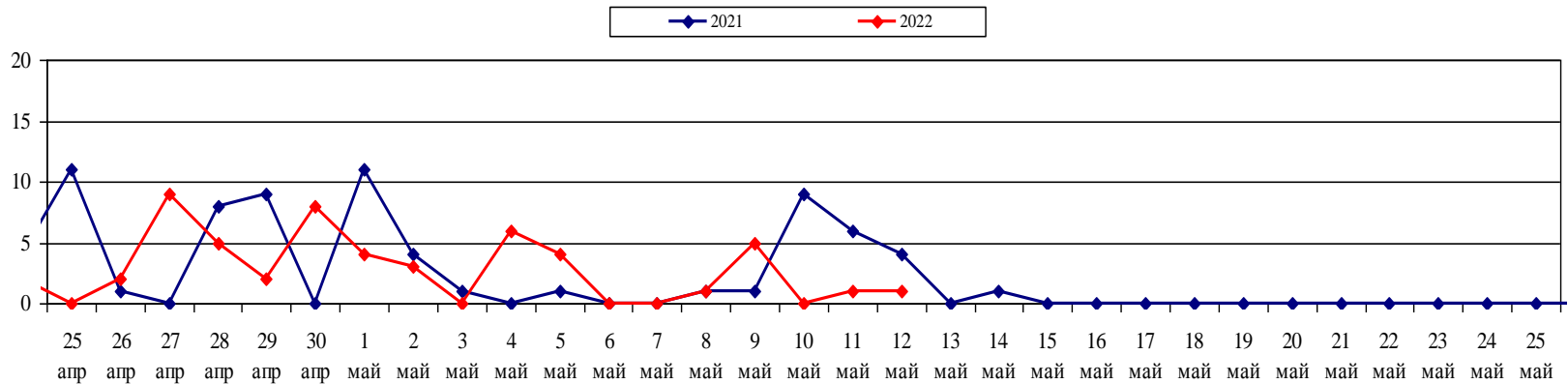
Площадь ландшафтных пожаров (2021-2022 гг., апрель - май)
