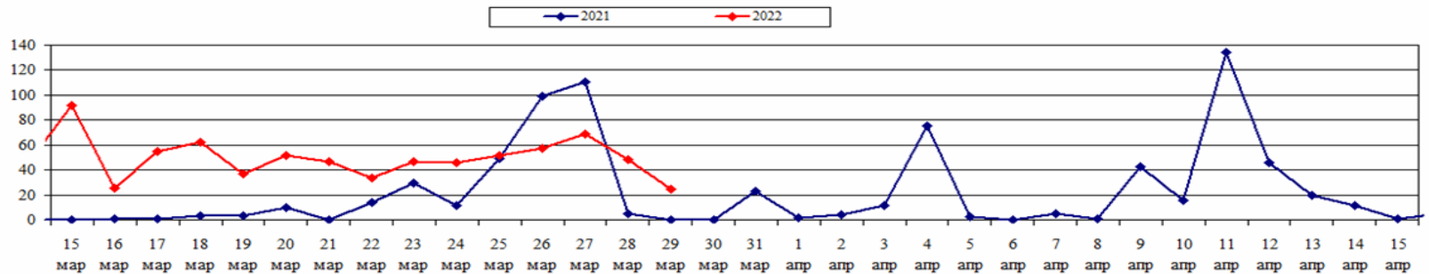
Площадь ландшафтных пожаров (2021-2022 гг., март-апрель)
