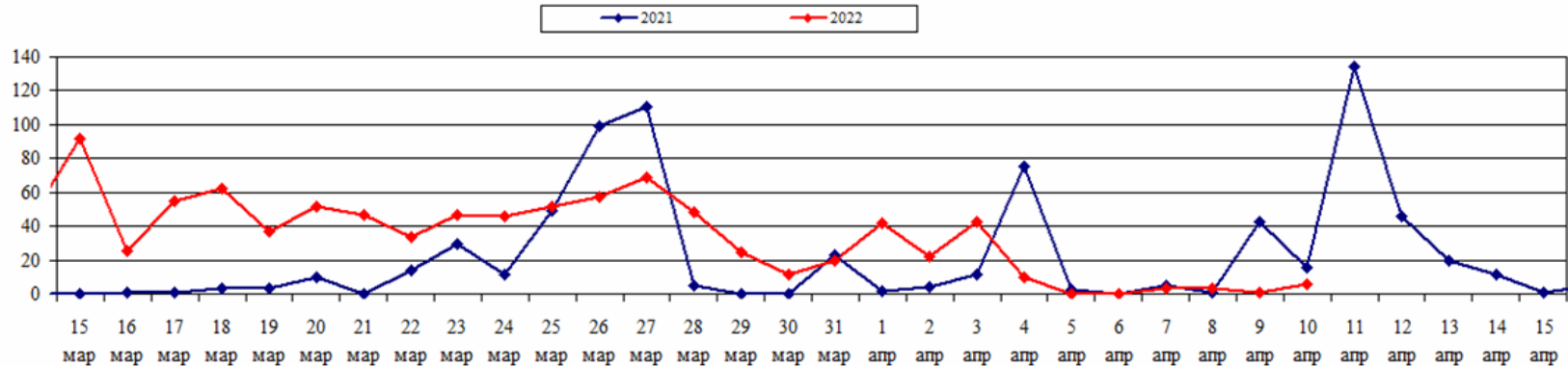
Площадь ландшафтных пожаров (2021-2022 гг., март-апрель)
