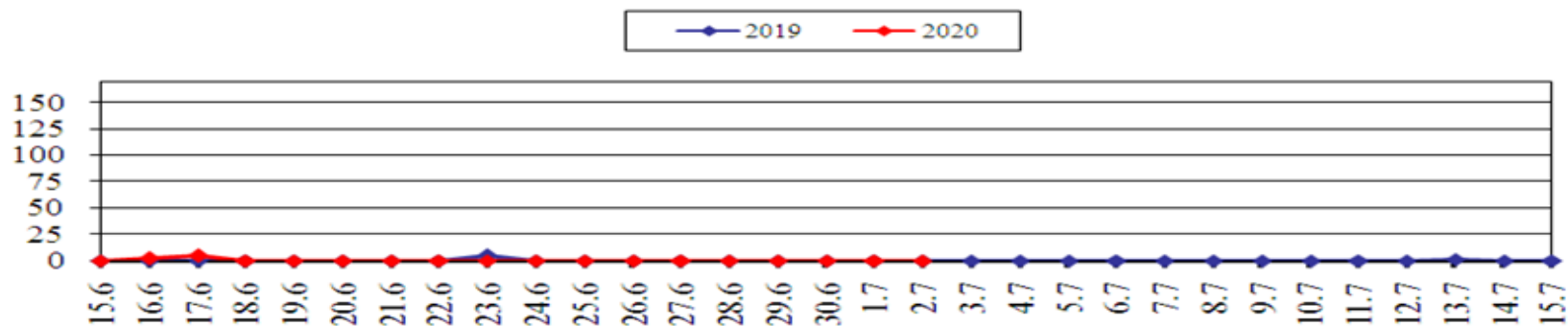
Площадь ландшафтных пожаров, га (2019; 2020 гг., июнь-июль)
