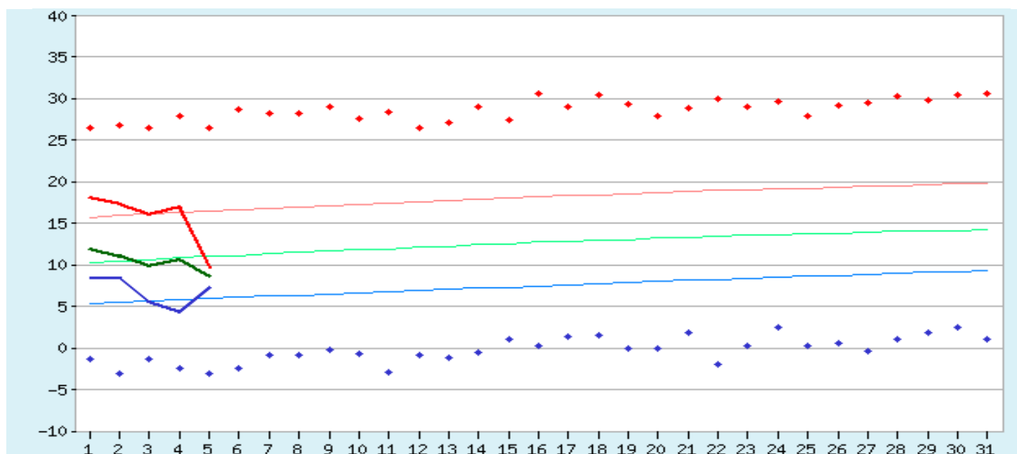
Температура воздуха в Калининграде. Май 2020 г.
