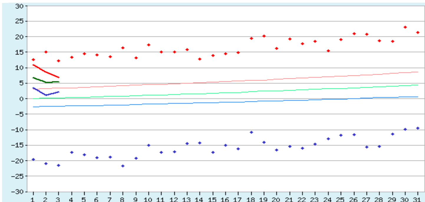
Температура воздуха в Калининграде. Март 2020 г.
