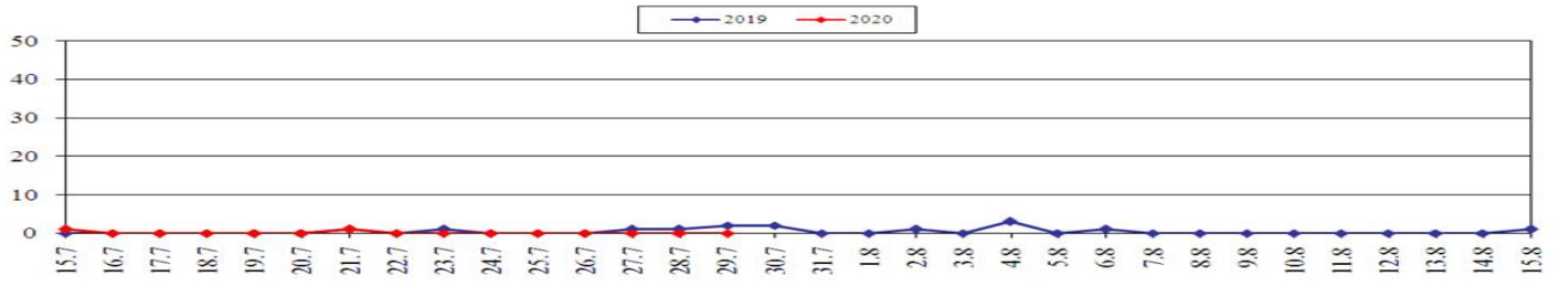
Площадь ландшафтных пожаров, га (2019; 2020 гг., июль-август)
