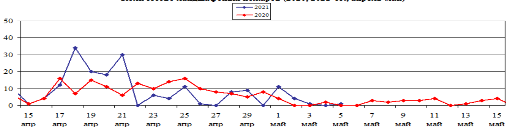
Площадь ландшафтных пожаров, га (2020; 2021 гг., апрель-май)
