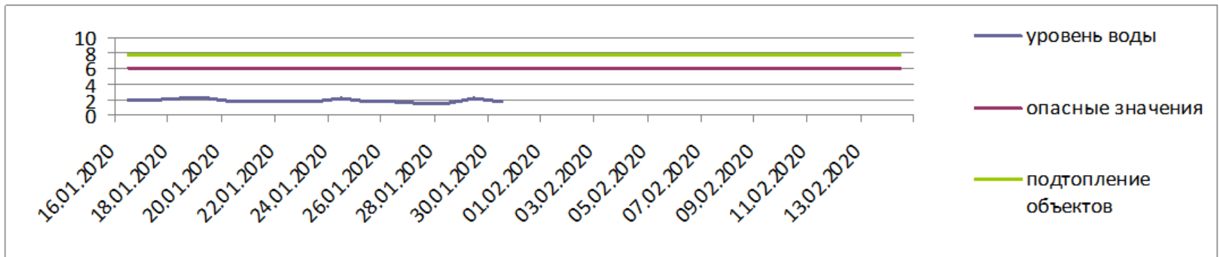
Уровень воды в р. Неман (м) (г. Смалнинкай, Литва)
