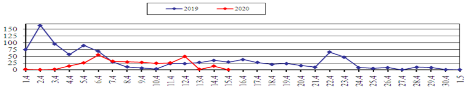
Площадь ландшафтных пожаров, га (2019; 2020 гг., апрель)
