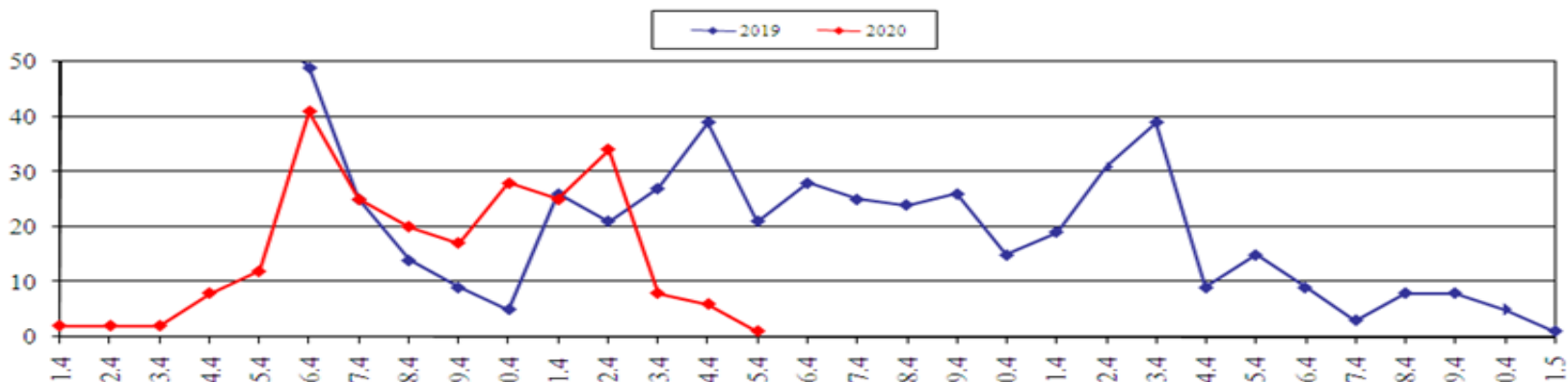
Количество ландшафтных пожаров (2019, 2020 гг., апрель)
