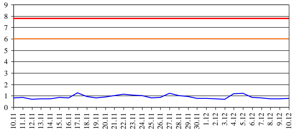
Уровень воды в р. Неман (г. Смалининкай, Литва)
