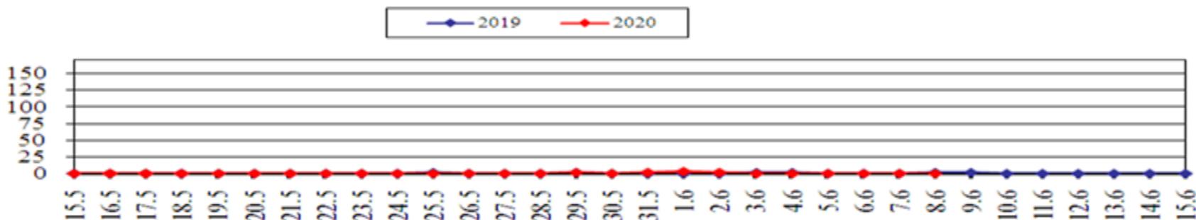
Площадь ландшафтных пожаров, га (2019; 2020 гг., май-июнь)
