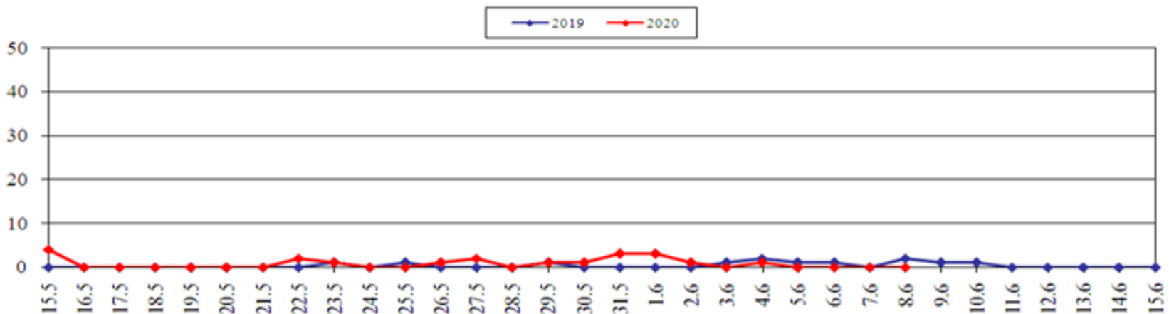
Количество ландшафтных пожаров (2019, 2020 гг., май-июнь)
