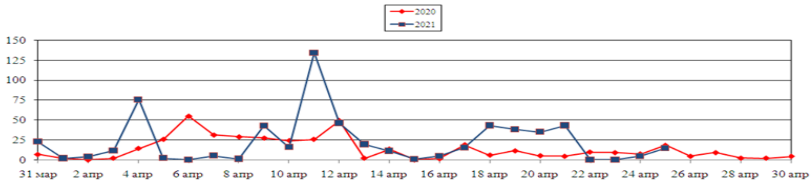
Площадь ландшафтных пожаров, га (2020; 2021 гг., апрель)
