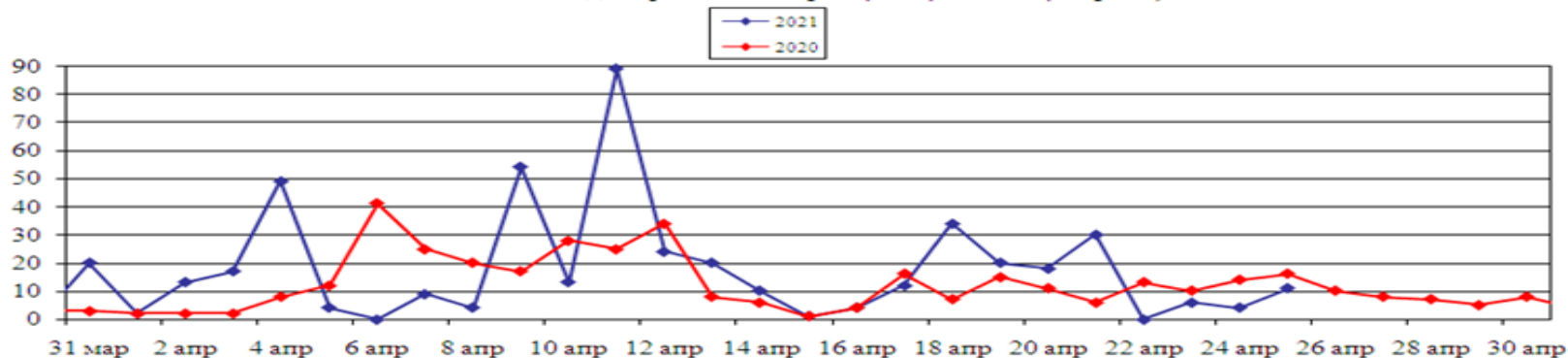
Количество ландшафтных пожаров (2020, 2021 гг., апрель)
