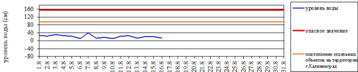
Уровень воды в р. Преголя относительно "0" поста МШК (г. Калининград)
