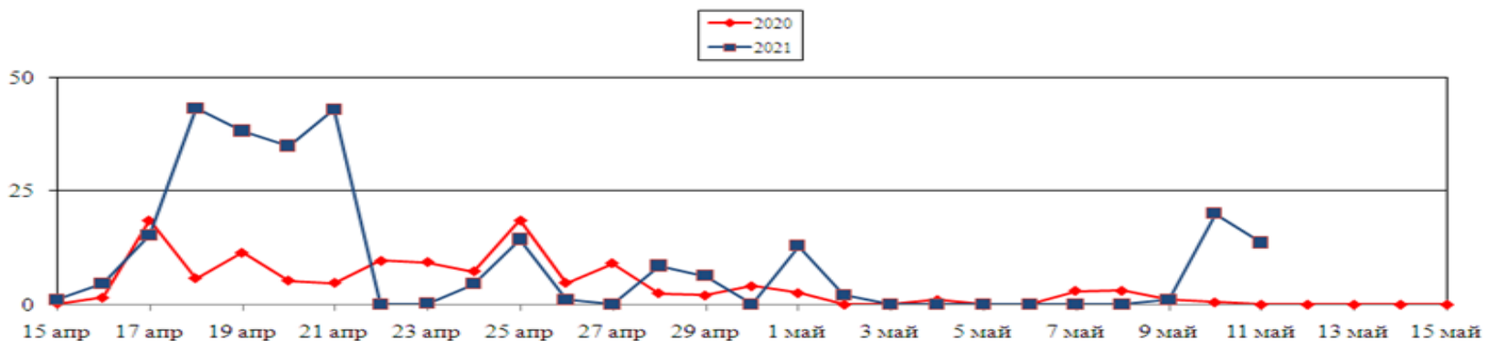
Площадь ландшафтных пожаров, га (2020; 2021 гг., апрель-май)
