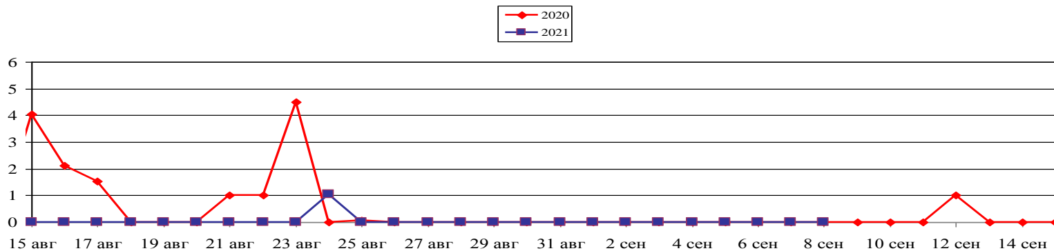
Площадь ландшафтных пожаров, га (2020; 2021 гг., август - сентябрь)
