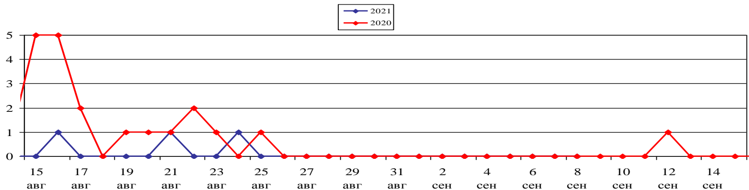
Количество ландшафтных пожаров (2020, 2021 гг., август - сентябрь)
