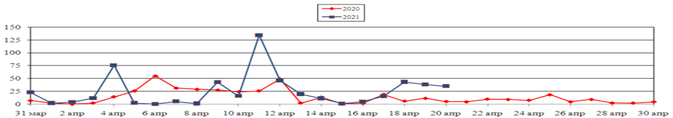
Площадь ландшафтных пожаров, га (2020; 2021 гг., апрель)
