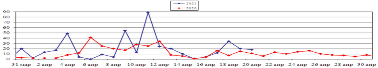
Площадь ландшафтных пожаров, га (2020; 2021 гг., апрель)
