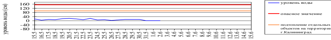
Уровень воды в р. Неман (г. Смалининкай, Литва)
