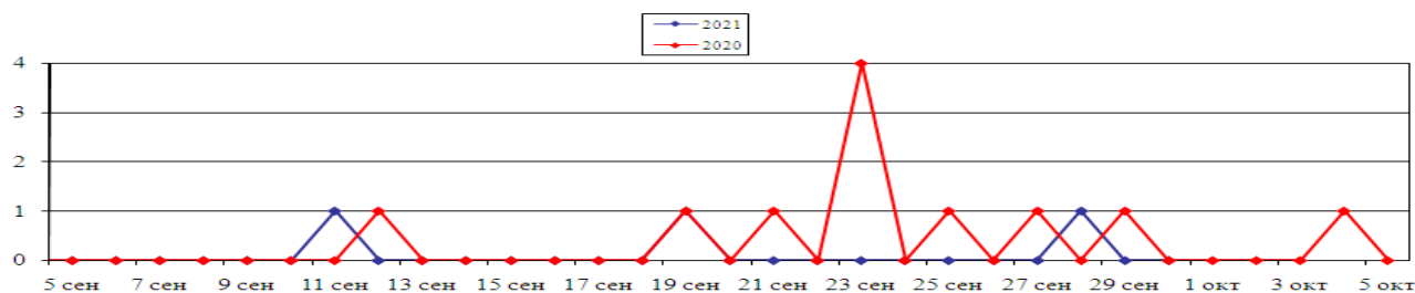
Площадь ландшафтных пожаров, га (2020; 2021 гг., сентябрь-октябрь)
