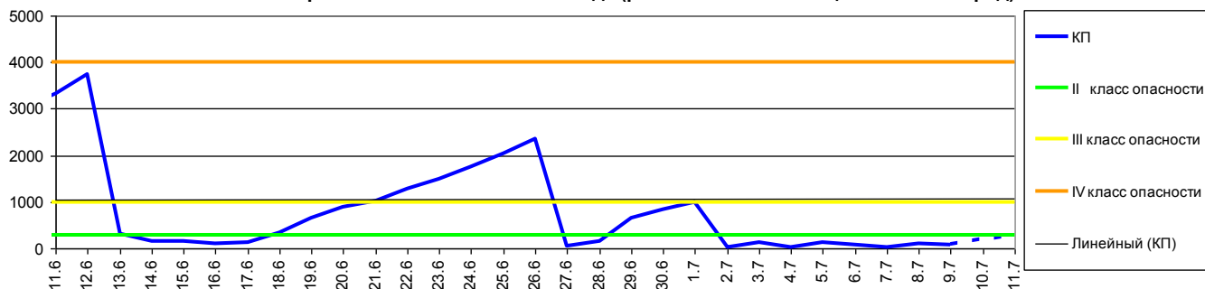
Комплексный показатель пожарной опасности лесов по условиям погоды за период с 11 июня по 09 июля и прогноз на 10-11 июля 2019 года (расчёт по метеостанции г.Калининград)
