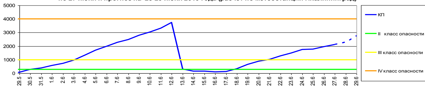
Комплексный показатель пожарной опасности лесов по условиям погоды за период с 29 мая по 27 июня и прогноз на 28-29 июня 2019 года (расчёт по метеостанции г.Калининград)
