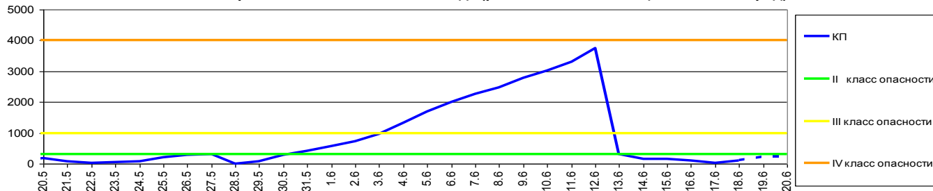
Комплексный показатель пожарной опасности лесов по условиям погоды за период с 20 мая по 18 июня и прогноз на 19-20 июня 2019 года (расчёт по метеостанции г.Калининград)
