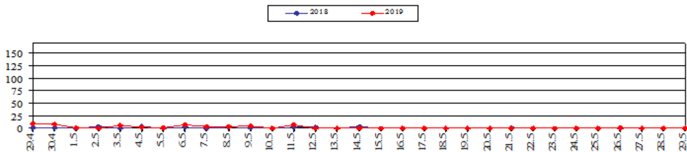
Площадь ландшафтных пожаров, га (2018, 2019 гг., апрель - май)
