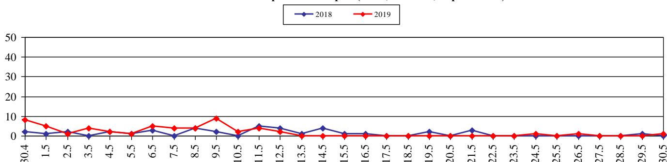
Количество ландшафтных пожаров (2018, 2019 гг., апрель-май)
