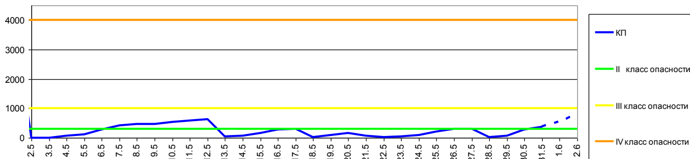
Комплексный показатель пожарной опасности лесов по условиям погоды за период с 2 мая по 31 мая и прогноз на 1-2 июня 2019 года (расчёт по метеостанции г.Калининград)
