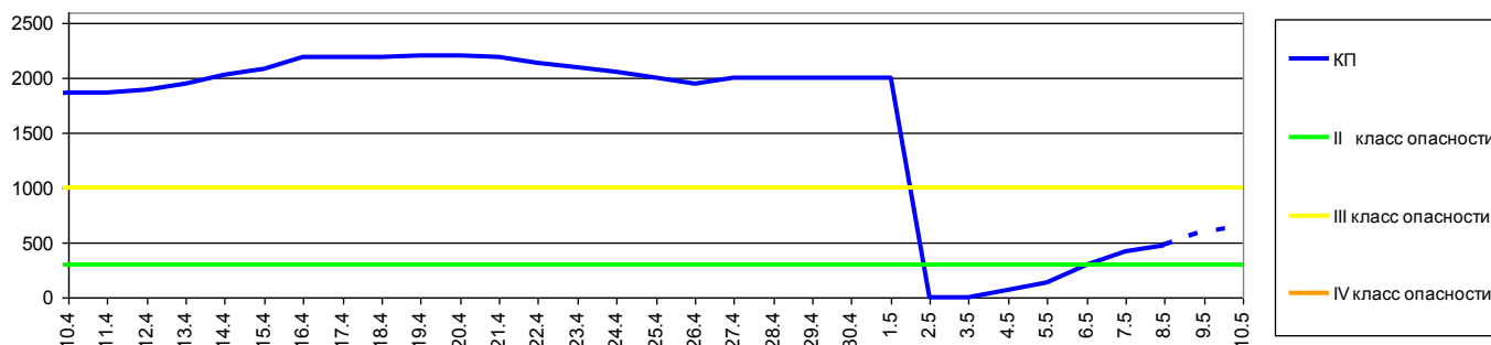
Комплексный показатель пожарной опасности лесов по условиям погоды за период с 10 апреля по 8 мая и прогноз на 9-10 мая 2019 года (расчёт по метеостанции г.Калининград)
