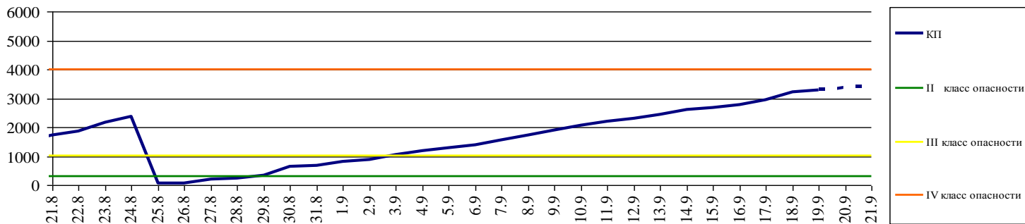
Комплексный показатель пожарной опасности лесов по условиям погоды за период с 21 августа по 19 сентября и прогноз на 20-21 сентября 2018 года (расчёт по метеостанции г.Калининград)
