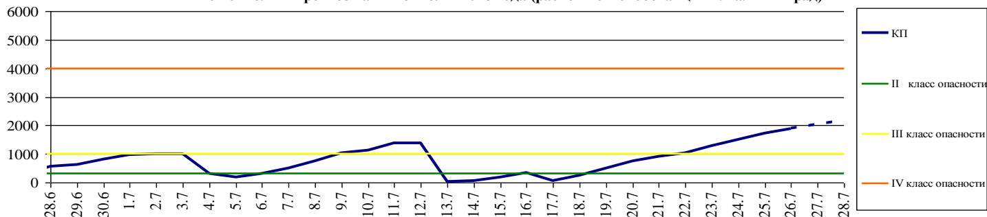
Комплексный показатель пожарной опасности лесов по условиям погоды за период с 28 июня по 26 июля и прогноз на 27-28 июля 2018 года (расчёт по метеостанции г.Калининград)
