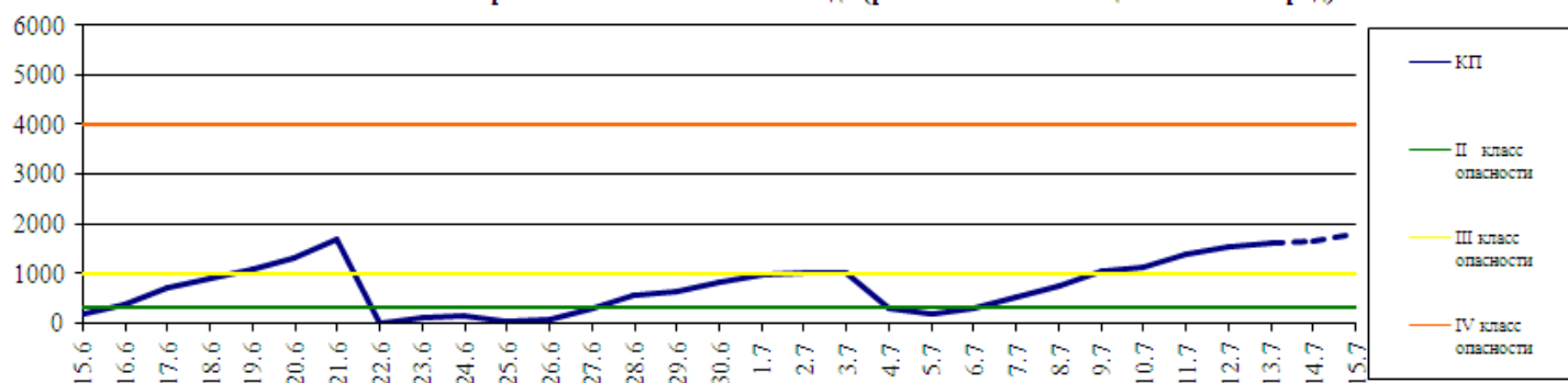
Комплексный показатель пожарной опасности лесов по условиям погоды за период с 15 июня по 13 июля и прогноз на 14-15 июля 2018 года (расчёт по метеостанции г.Калининград)
