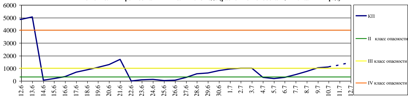
Комплексный показатель пожарной опасности лесов по условиям погоды за период с 12 июня по 10 июля и прогноз на 11-12 июля 2018 года (расчёт по метеостанции г.Калининград)
