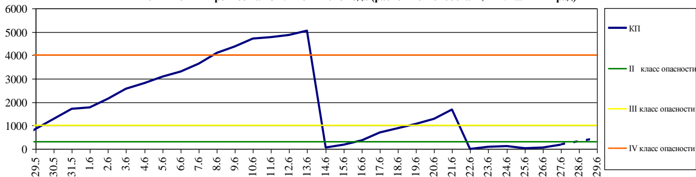
Комплексный показатель пожарной опасности лесов по условиям погоды за период с 29 мая по 27 июня и прогноз на 28-29 июня 2018 года (расчёт по метеостанции г.Калининград)
