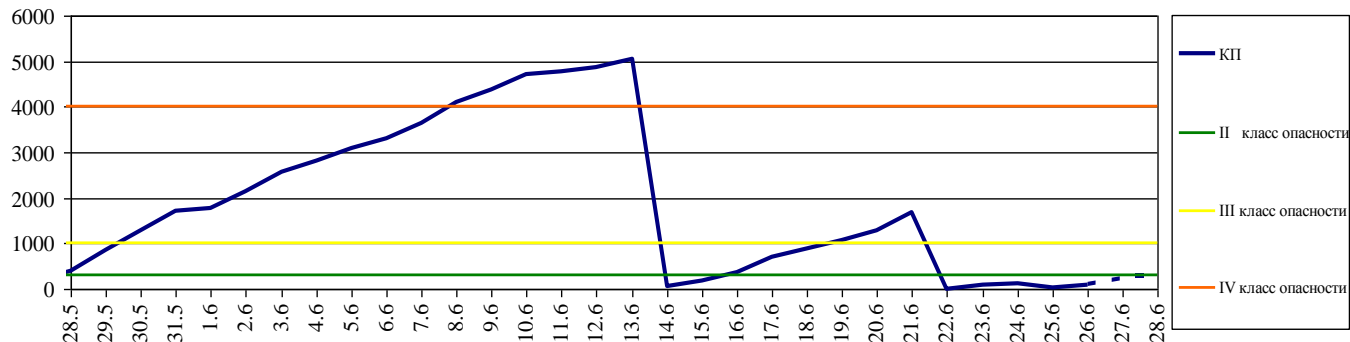
Комплексный показатель пожарной опасности лесов по условиям погоды за период с 28 мая по 26 июня и прогноз на 27-28 июня 2018 года (расчёт по метеостанции г.Калининград)
