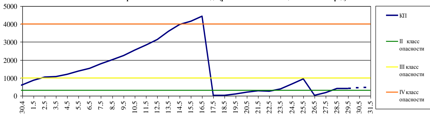
Комплексный показатель пожарной опасности лесов по условиям погоды за период с 30 апреля по 29 мая и прогноз на 30-31 мая 2018 года (расчёт по метеостанции г.Калининград)
