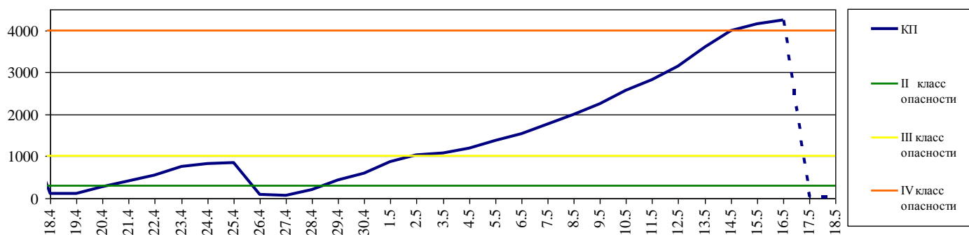
Комплексный показатель пожарной опасности лесов по условиям погоды за период с 18 апреля по 15 мая и прогноз на 16-18 мая 2018 года (расчёт по метеостанции г.Калининград)
