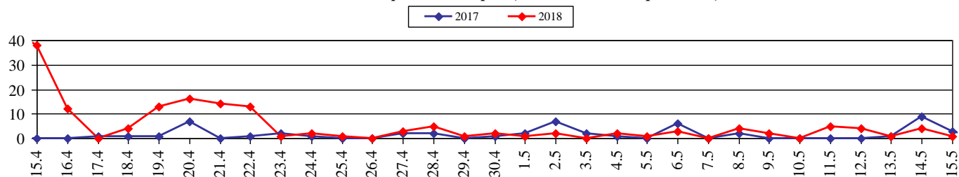
Площадь ландшафтных пожаров, га (2017, 2018 гг., апрель- май)
